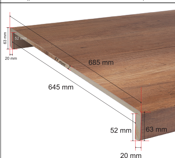
DOPPELStufe für gewendelte Treppen (passend für Stufen ab 31 cm Tiefe)
