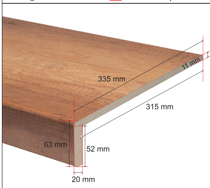
EINZELStufe für geradläufige Treppen (passend für Stufen bis 31 cm Tiefe)
